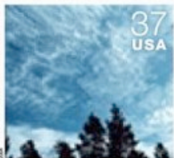
Cirrocumulus undulatus
