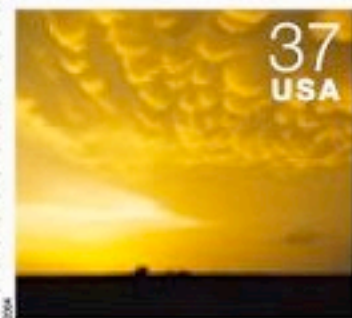
Cumulonimbus mammatus
